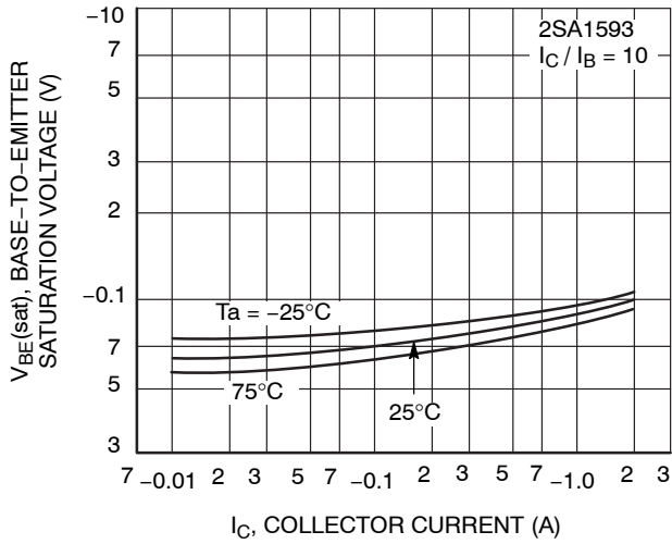
Figure 14. V_{BE(sat)} - I_C
